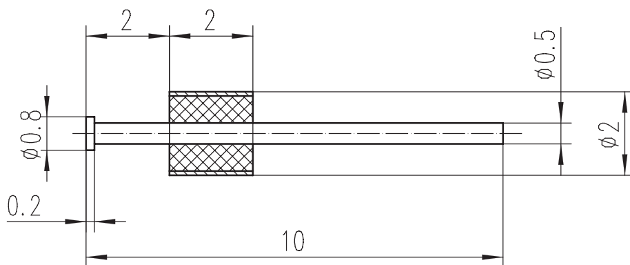
型 号 PT202050-10/2
